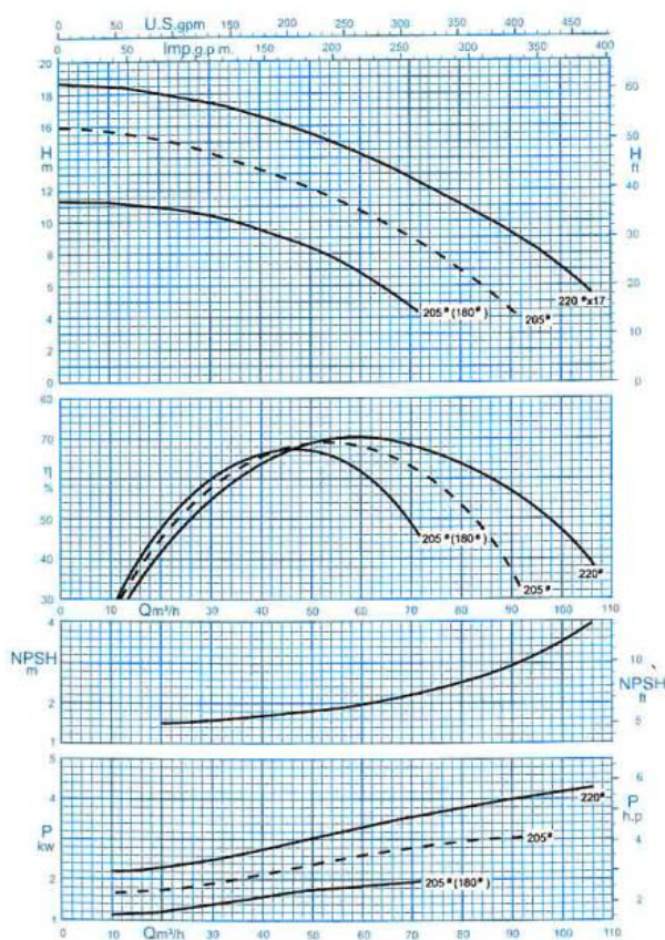
دور موتور ۱۴۵۰ / 1450 rpm منحني يك طبقه / For 1 Stage
